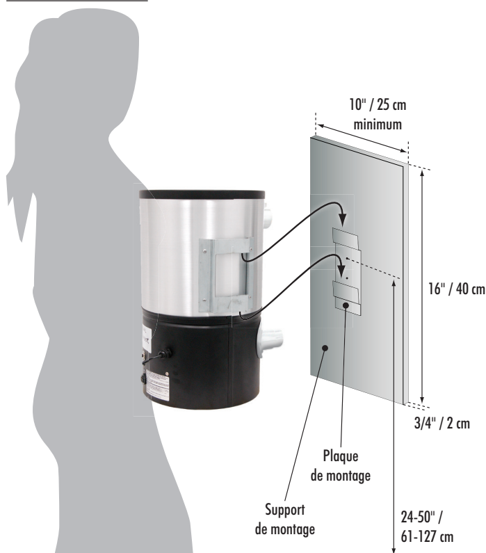
Fig.1 Installation de l'unité motrice au mur.
